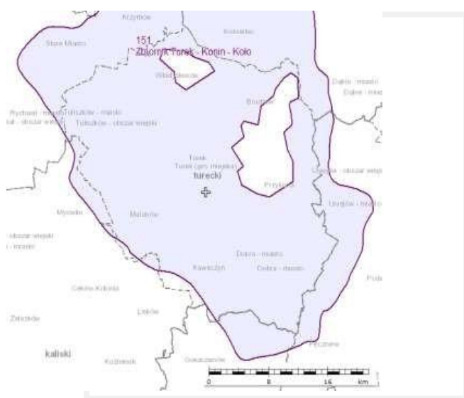
Rysunek 7 Główny zbiornik wód podziemnych na terenie powiatu tureckiego.
