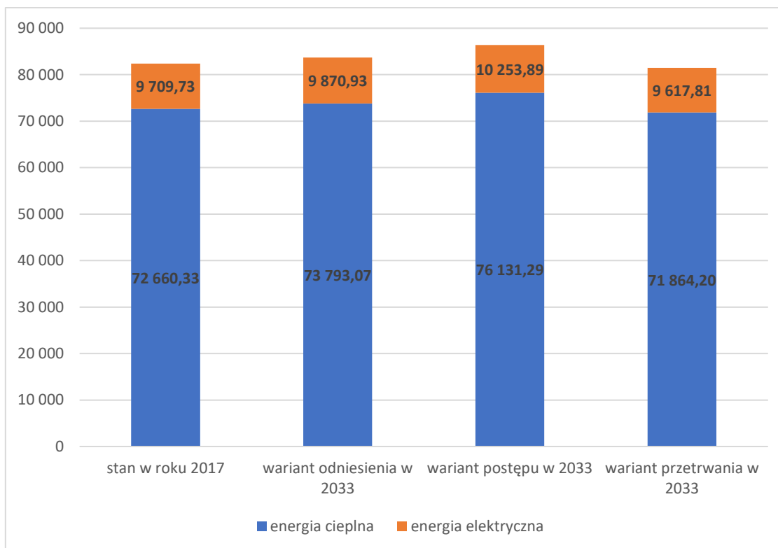
Rysunek 4 Prognoza zużycia energii w MWh/rok dla gminy i miasta Tuliszków.
